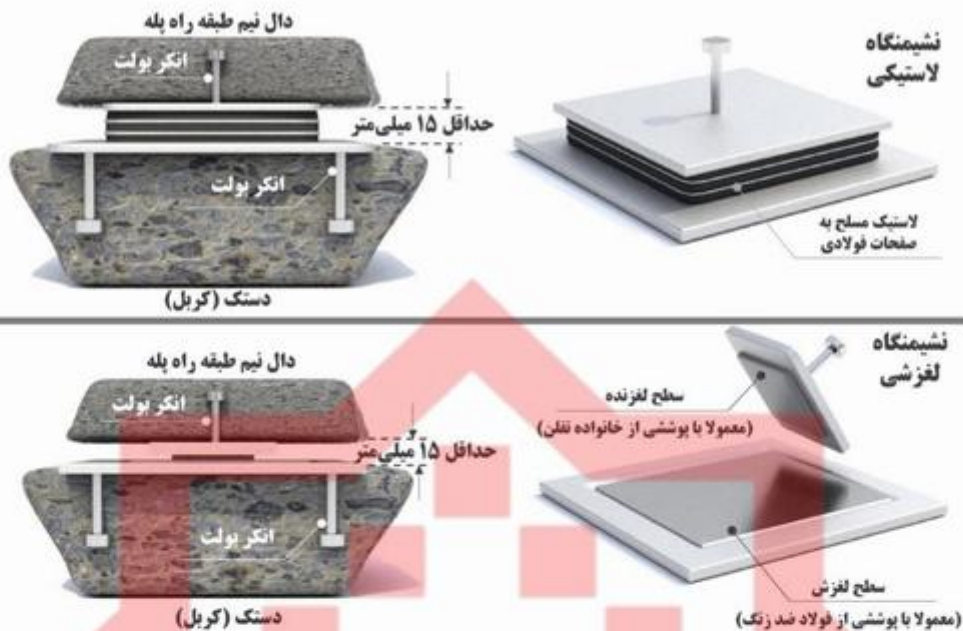
شکل ۴-۳۷ نمونه‌ای از جزئیات نشیمگاه‌های لاستیکی و لغزشی به منظور جداسازی راه پله
