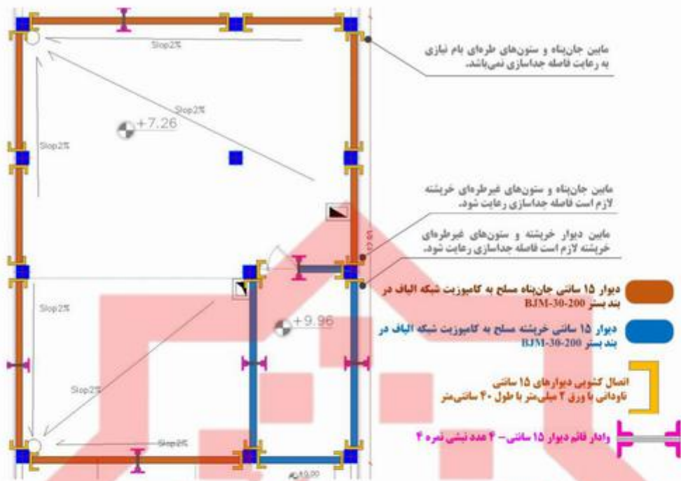
شکل پ-۱۰- تیپ‌بندی دیوارها، جانمایی و ادارهای قائم و اتصالات کشویی در بام و خرپشته
