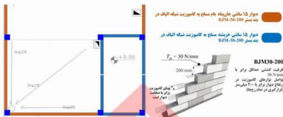
شکل پ-۴-۶ تیپ بندی دیوارهای جان پناه بام و خرپشته (ستون‌ها به اندازه ارتفاع جان پناه از کف بام امتداد یافته است. در محل خرپشته، ستون‌ها تا سقف خرپشته امتداد دارند).
