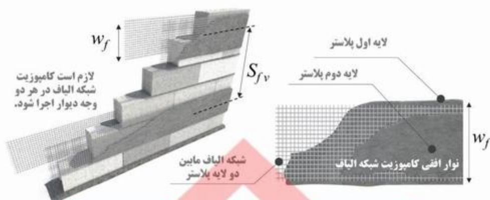
شکل ۴-۳ کمیت‌های مورد نیاز برای محاسبه ظرفیت خمش افقی دیوارهای بنایی مسلح به کامپوزیت شبکه الیاف به صورت نوارهای افقی.
