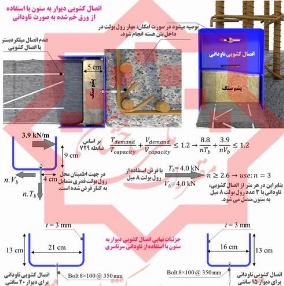
شکل پ-۱۹ جزئیات نهایی اتصال دیوار به ستون به صورت ناودانی سراسری
