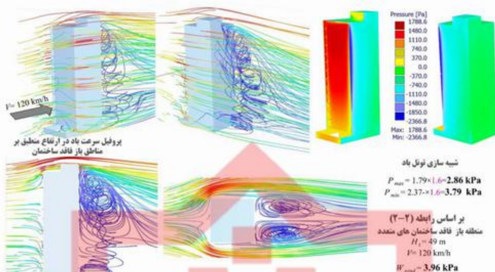
شکل پ-۲ بررسی دقت رابطه (۲-۲) در تخمین فشار/ مکش ناشی از باد برای یک ساختمان ۱۴ طبقه به ارتفاع ۴۹ متر واقع در منطقه‌ای فاقد ساختمان‌های متعدد و سرعت باد مبنای ۱۲۰ کیلومتر بر ساعت.
