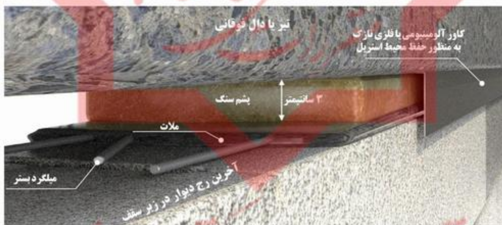
شکل پ-۱۷ اجرای ملات و میلگرد بستر در آخرین رج دیوار در زیر سقف - اجرای میلگرد بستر در آخرین رج الزامی نبوده اما قابل توصیه است.
