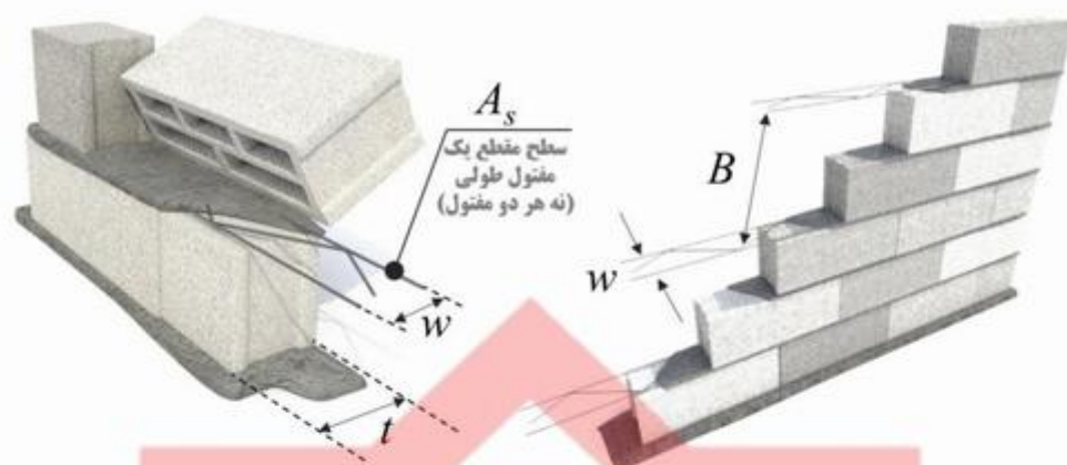
شکل ۲-۳ کمیت‌های مورد نیاز برای محاسبه ظرفیت خمشی افقی دیوارهای بتابی مسلح به میلگرد بستر.
