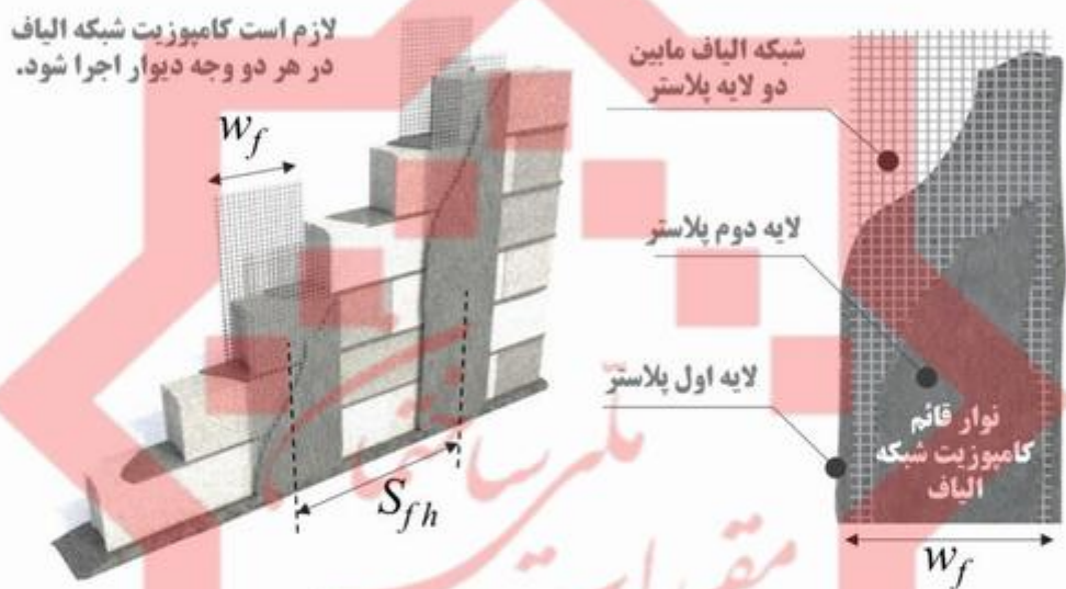
شکل ۵-۳ کمیت‌های مورد نیاز برای محاسبه ظرفیت خمشی قائم دیوارهای بنایی مسلح به کامپوزیت شبکه الیاف به صورت نوارهای قائم.
