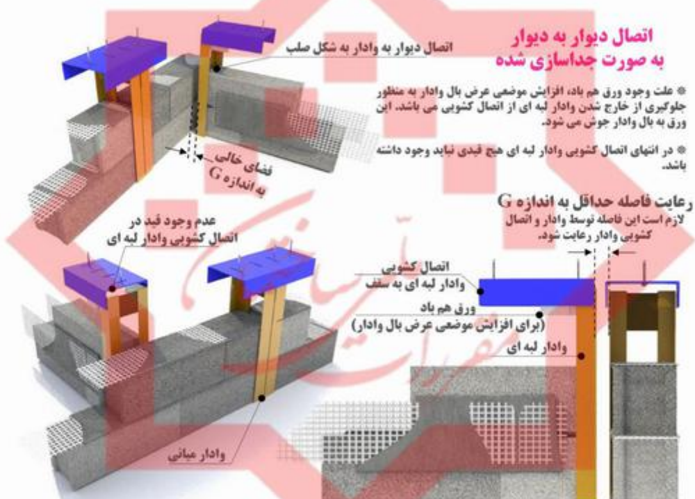
شکل ۴-۱۲ اتصال دیوار به دیوار به‌صورت جداسازی شده.
