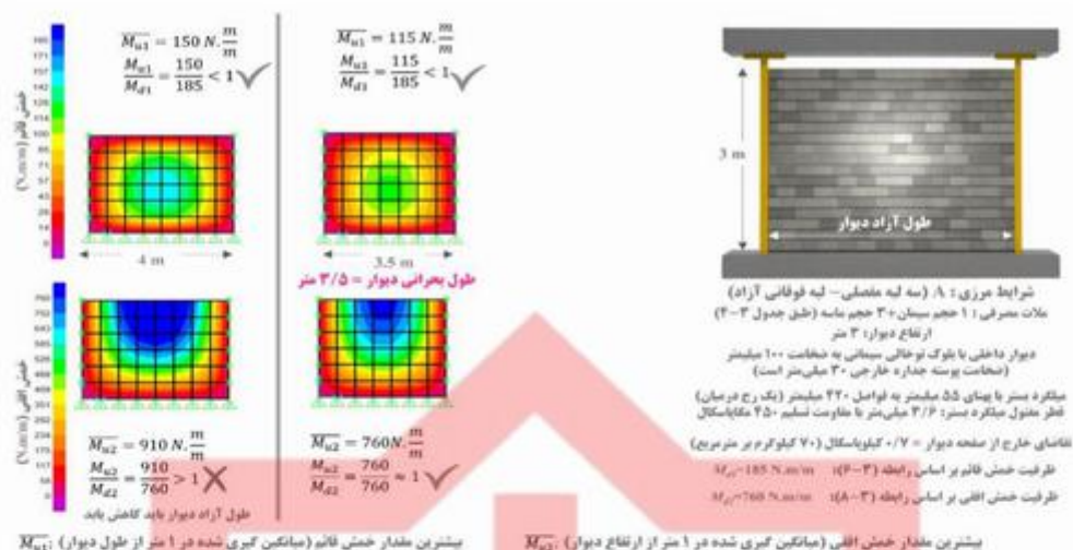
شکل ۹-۳ نمونه روند محاسبه طول بحرانی برای دیواری با شرایط مرزی از نوع A (سه لبه مفصل - لبه فوقانی آزاد) - با استفاده از تحلیل اجزاء محدود.
